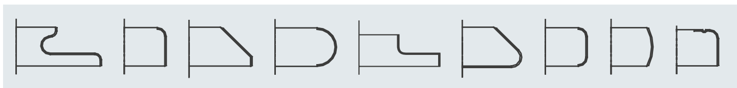
Profilo J su pannelli MDF e truciolare con bordi in PVC fino a 0,6 mm di spessore, ABS, e PP
