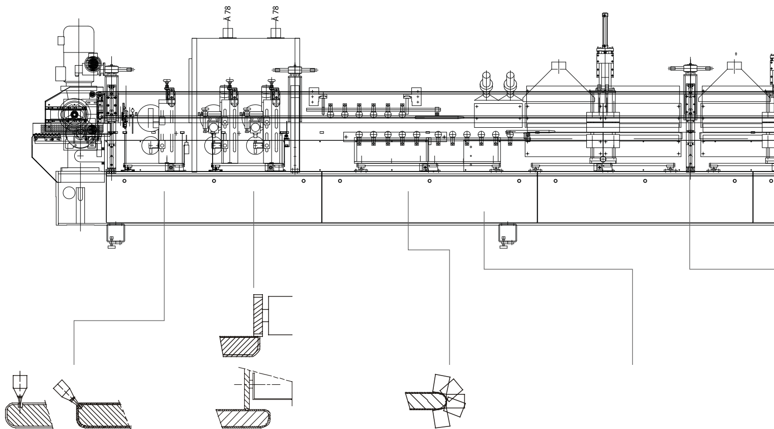
Zona sigillatura giunzione
