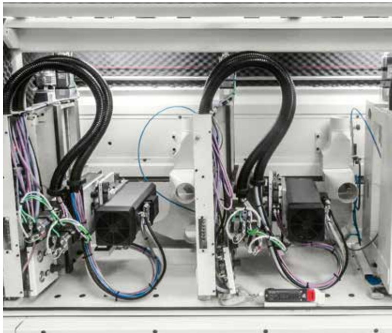
Composizione zona a profilare multi utensile per la lavorazione di differenti profili.
