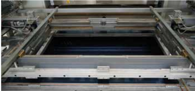
Cornice prelastra automatica: sistema di regolazione completamente automatico con traverse telescopiche. Garantisce a copertura di tutte le misure senza nessun attrezzaggio manuale garantendo sempre la massima tenuta della lastra.
