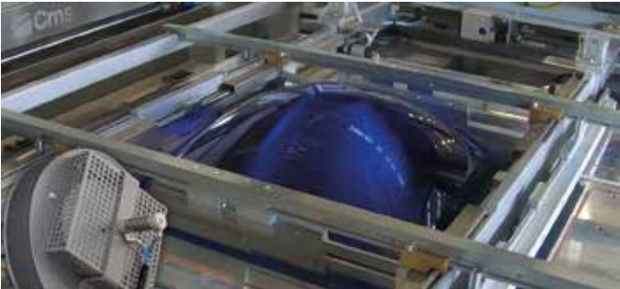
Sistema elettronico di imbutitura lastra: la funzione di imbutitura viene realizzata tramite un ventilatore controllato elettronicamente. Il controllo dell'altezza imbutitura è effettuato con sensore laser, infrarosso o ad ultrasuoni.
