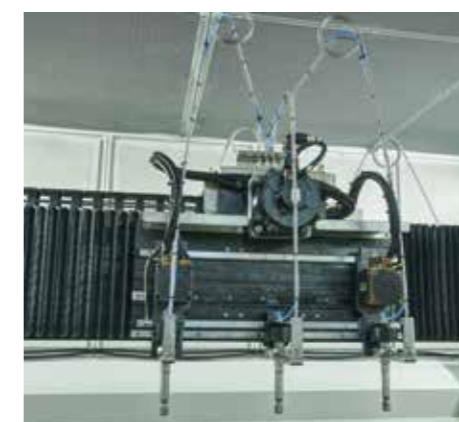
РЕЖУЩИЕ ГОЛОВКИ Дополнительные головки для резки чистой водой, состоящие из тележек по 3 до 5 головок каждая.
