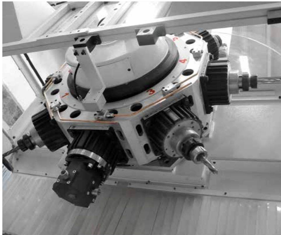
R8 Nouvelle unité opérationnelle revolver avec 8 mandrins de caractéristiques différentes et une puissance allant jusqu'à 8,5 kW. Elle se caractérise par un changement d'outil extrêmement rapide, sa solidité et sa fiabilité.
