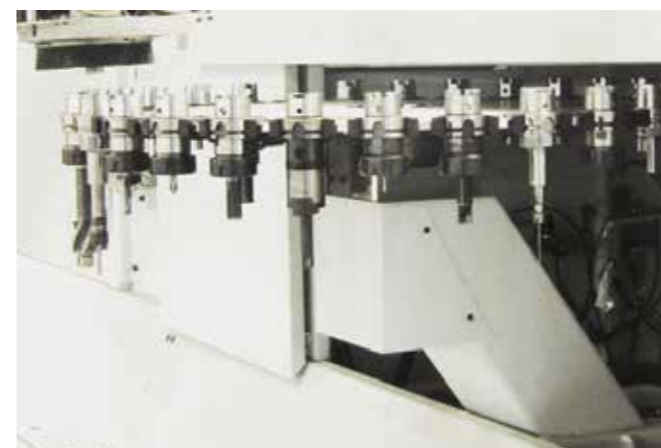
Depósito porta ferramentas giratório automático com 30 estações
